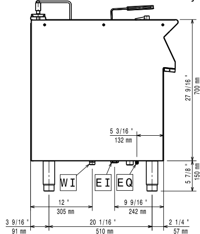
Zij aanzicht
