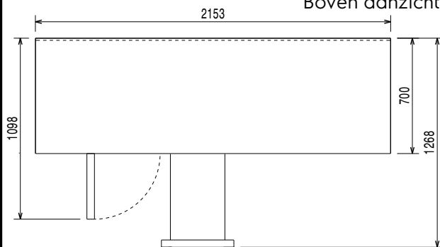
Boven aanzicht
