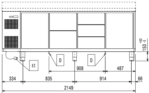
Zij aanzicht
