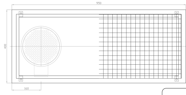
Boven aanzicht
