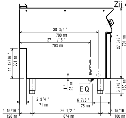
Zij aanzicht
